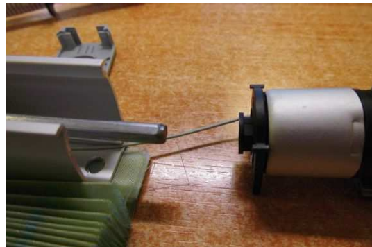
↑ 4. (Kun hvis kædetrækket er svært at betjene). Tag kædetrækket ud og indsæt korrekt i røret.
